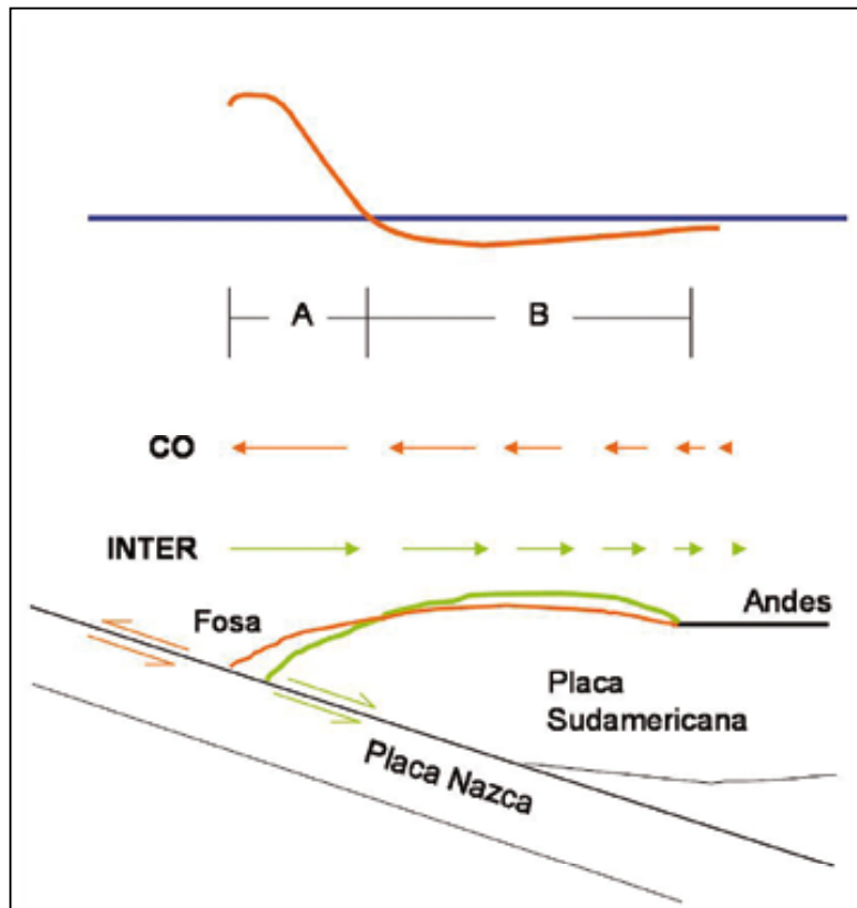
Figura 4. Movimientos cosísmicos, durante el intersísmico se forma la flexura antiforme (verde), ambas placas están acopladas y se mueven hacia la Cordillera de Los Andes. Durante el cosísmico (rojo) las placas se desacoplan, la Placa Sudamericana se mueve hacia la fosa generándose una zona de alzamiento mas cerca de la fosa y una zona de subsidencia más lejos en dirección hacia la cordillera como ilustra la curva superior correspondiente a los movimientos cosísmicos verticales.
